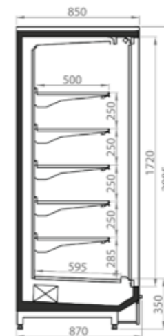
MEDUSA Montenegro Doors
