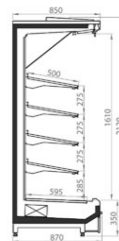
MEDUSA Montenegro AC FV
